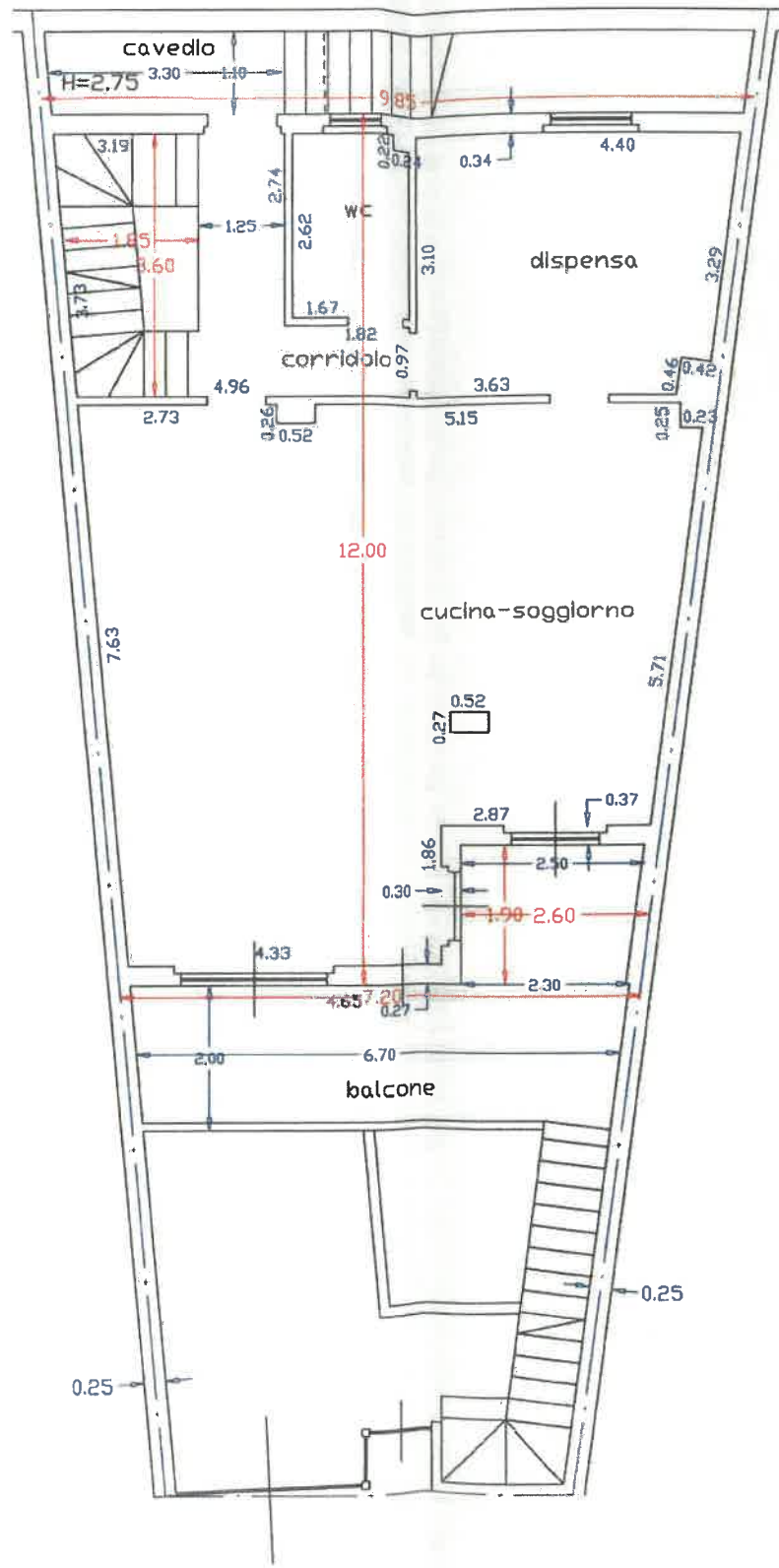
PIANO SEMINTERRATO h(grezzo) >> m. 2,70
