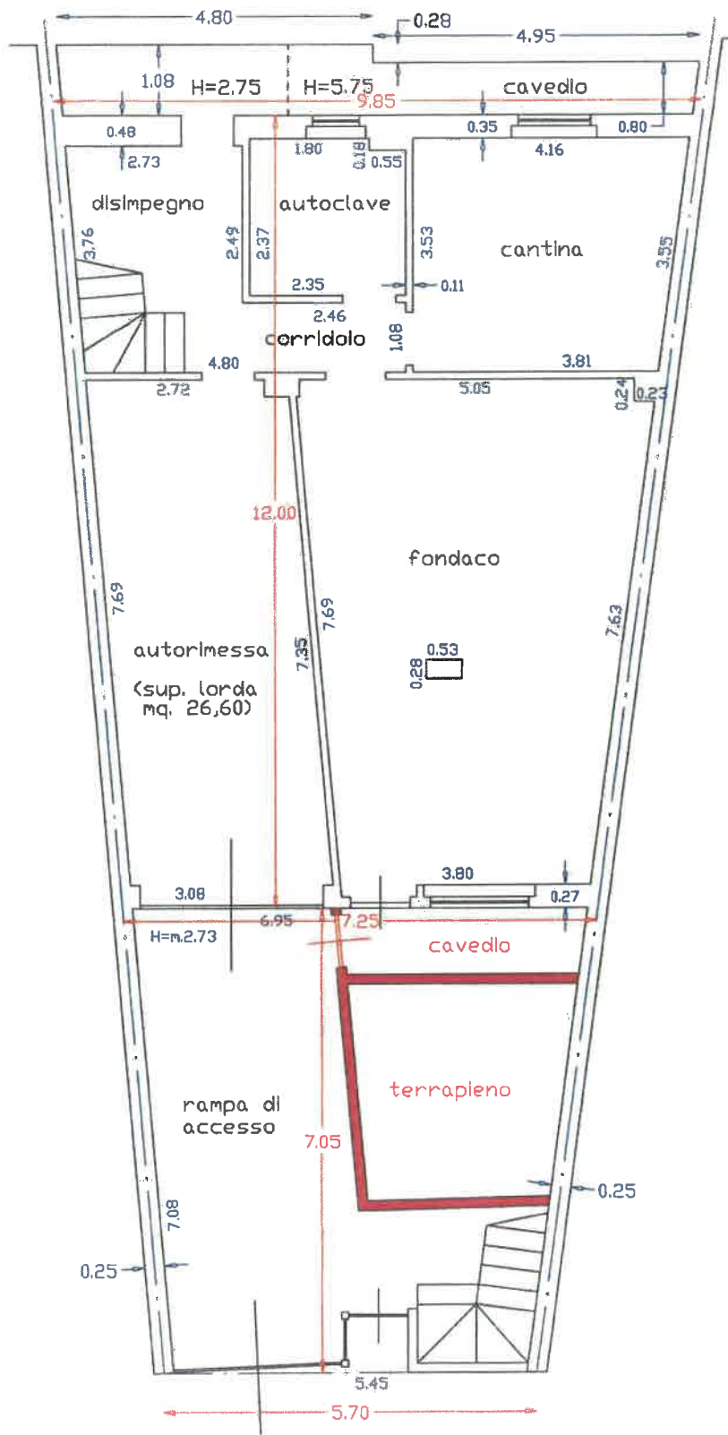
PIANO INTERRATO h(grezzo) >> m. 2,70
