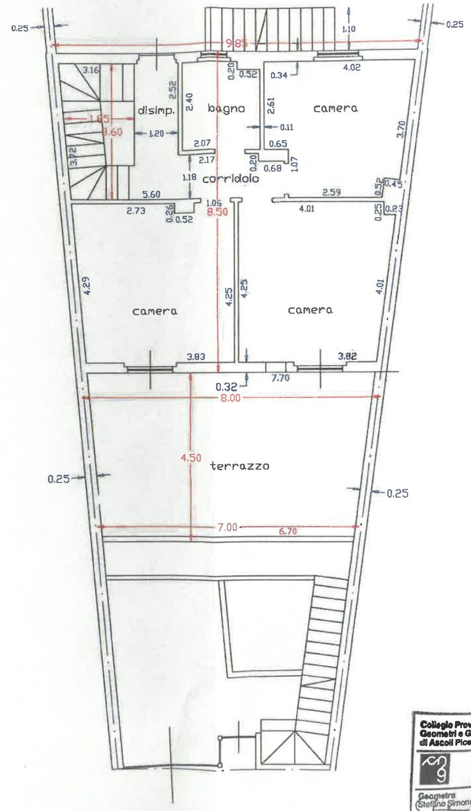
PIANO TERRA h(grezzo) >> m. 2,70
